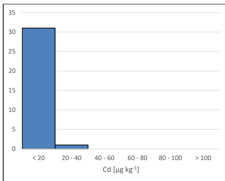
Rys. 2 Rozkład stężeń kadmu w badanych próbkach kukurydzy.
