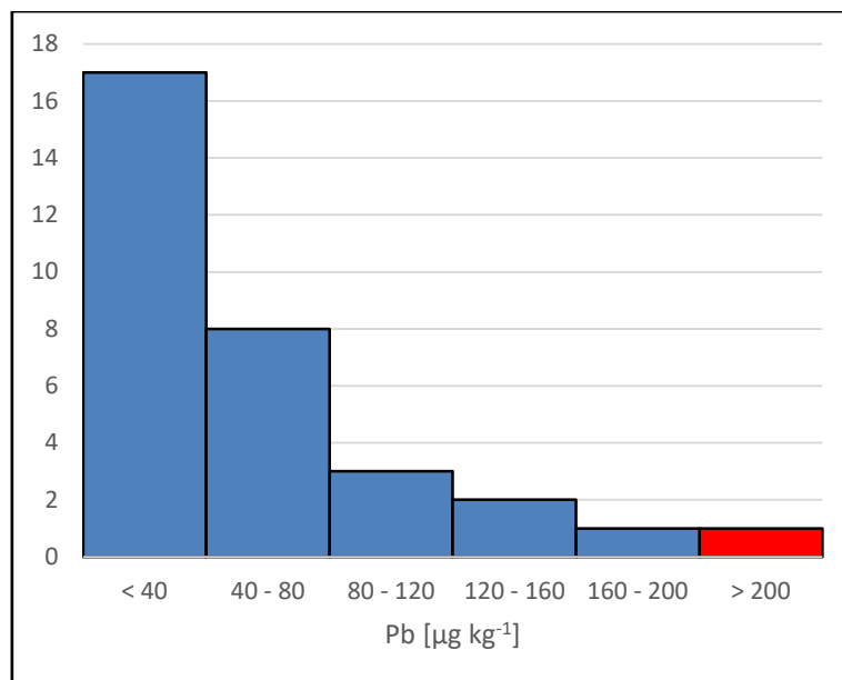
Rys. 1 Rozkład stężeń ołowiu w badanych próbkach kukurydzy.
