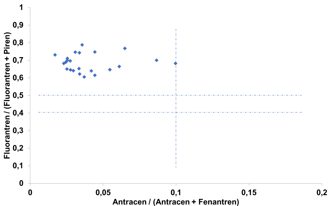
Rys. 2 Rozkład wartości diagnostycznych dla stężeń węglowodorów aromatycznych w ziarnie pszenżyta.
