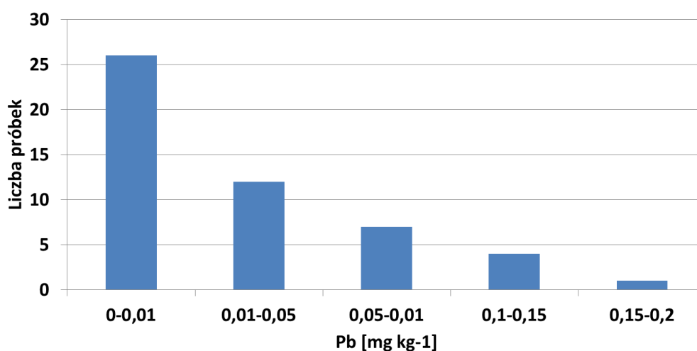
Rys. 3 Rozkład stężeń ołowiu w badanych próbkach pszenżyta.
