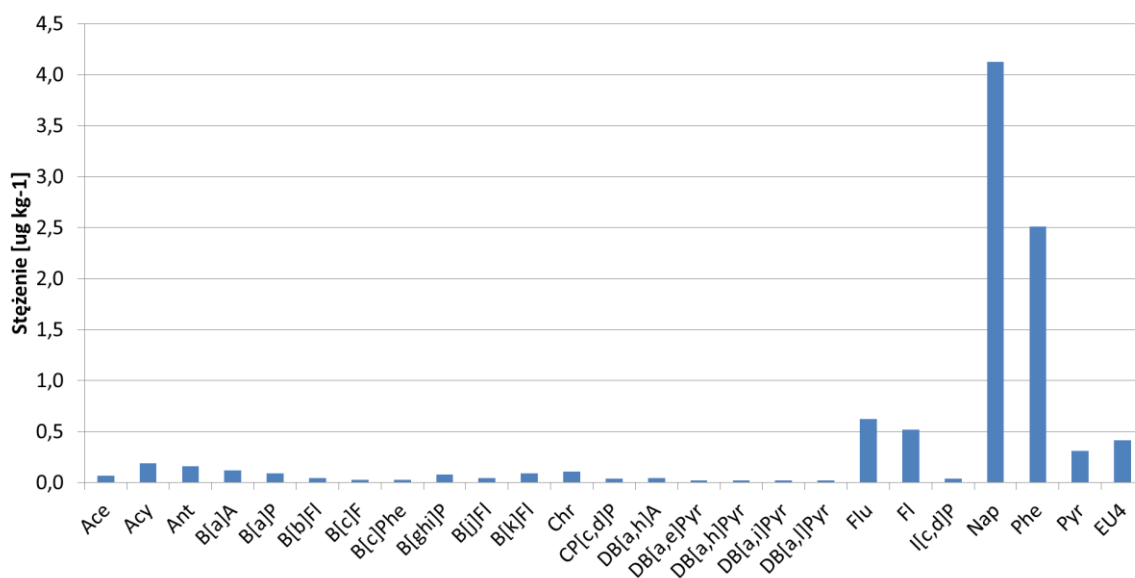
Rys 1. Profil w\u0119glowodor\u00f3w aromatycznych w ziarnie pszen\u017cyta.
