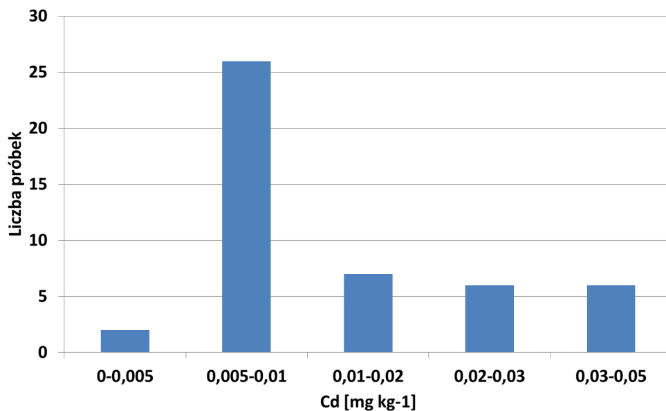
Rys. 4 Rozkład stężeń kadmu w badanych próbkach pszenżyta.
